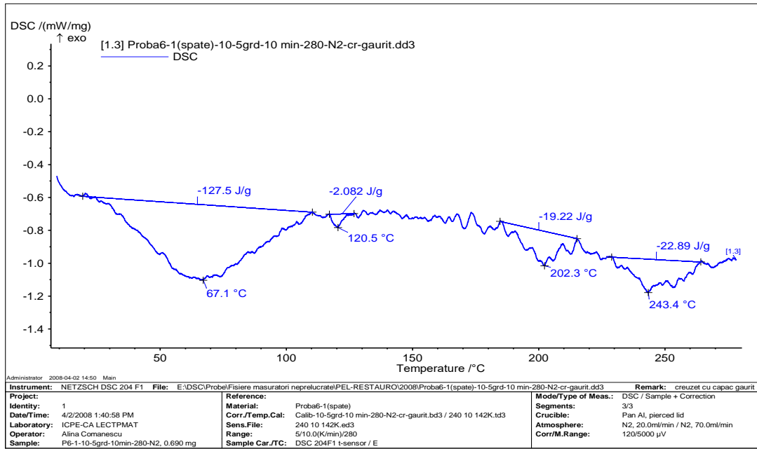
Fig. 1.14. Curba DSC pentru proba de piele P6-1
