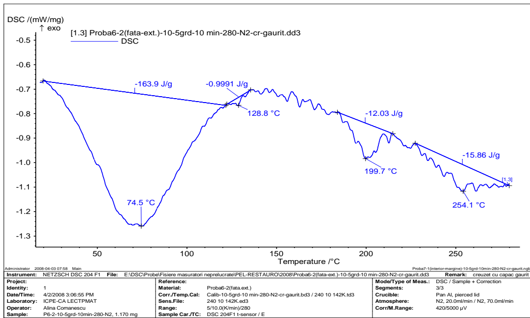
Fig. 1.15. Curba DSC pentru proba de piele P6-2
